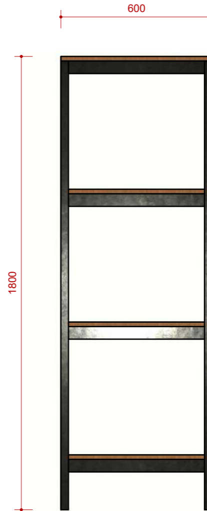
ELEVAÇÃO LATERAL ESCALA 1:15
