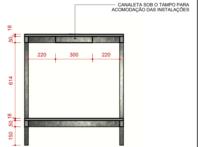
CORTE A ESCALA 1:20
