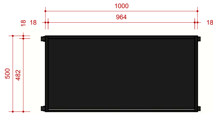
VISTA DE TOPO ESCALA 1:15
