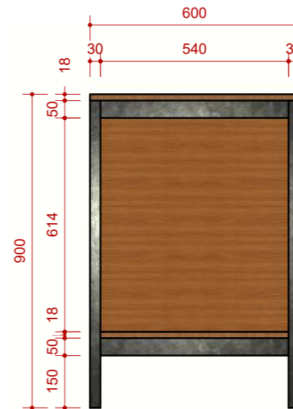
ELEVAÇÃO LATERAL ESCALA 1:15
