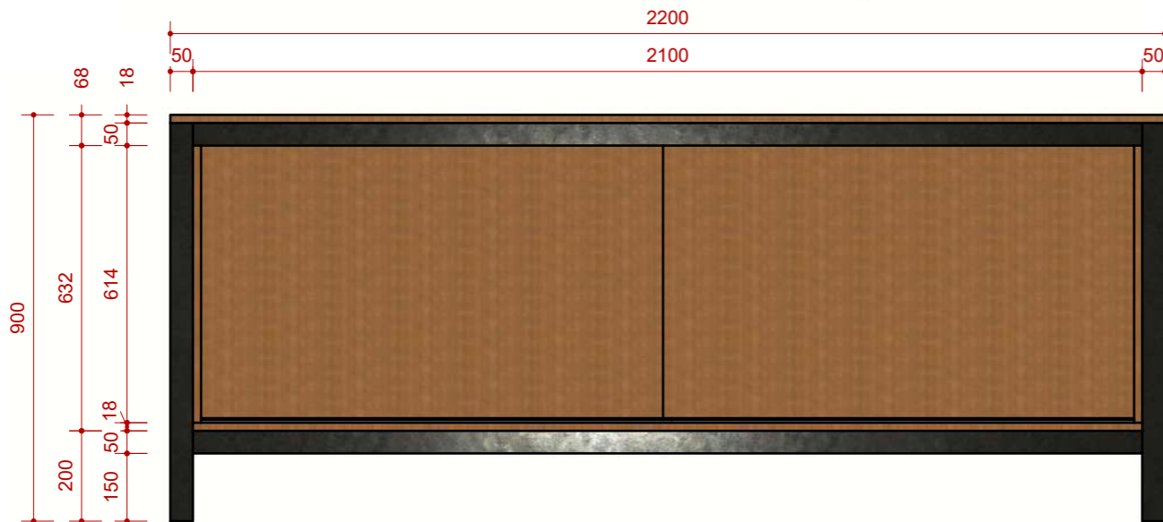
ELEVAÇÃO FRONTAL ESCALA 1:15
