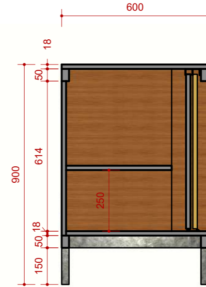
CORTE A ESCALA 1:20
