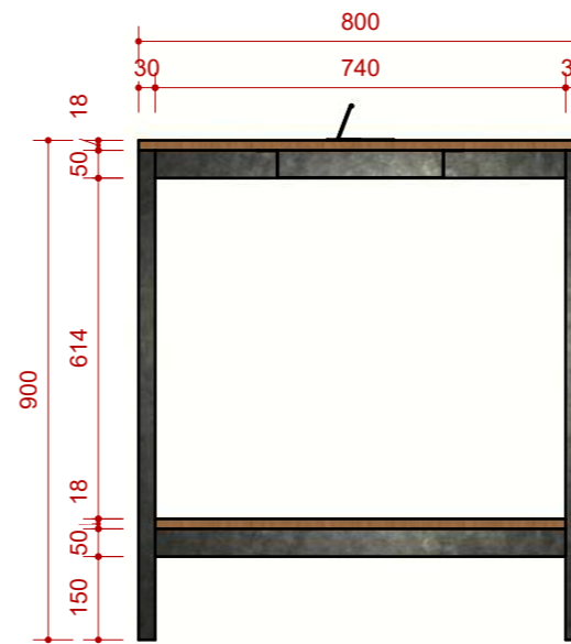
ELEVÇÃO LATERAL ESCALA 1:15
