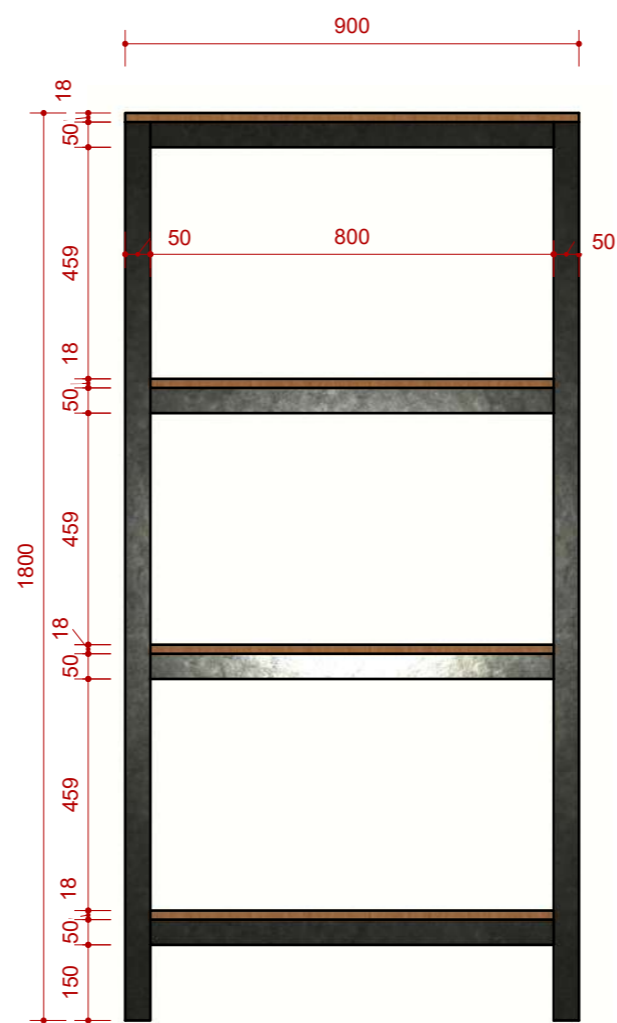
ELEVAÇÃO FRONTAL ESCALA 1:15
