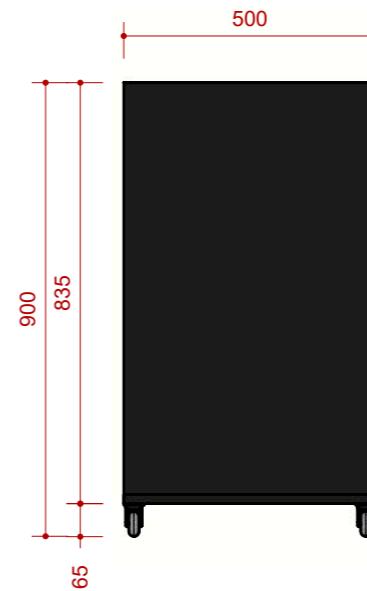
ELEVAÇÃO LATERAL ESCALA 1:15
