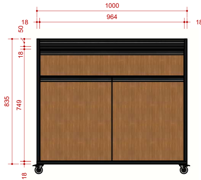
ELEVAÇÃO FRONTAL ESCALA 1:15
