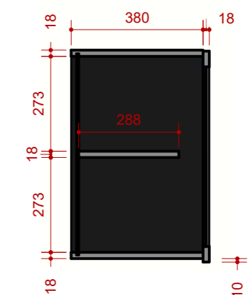
CORTE A ESCALA 1:20
