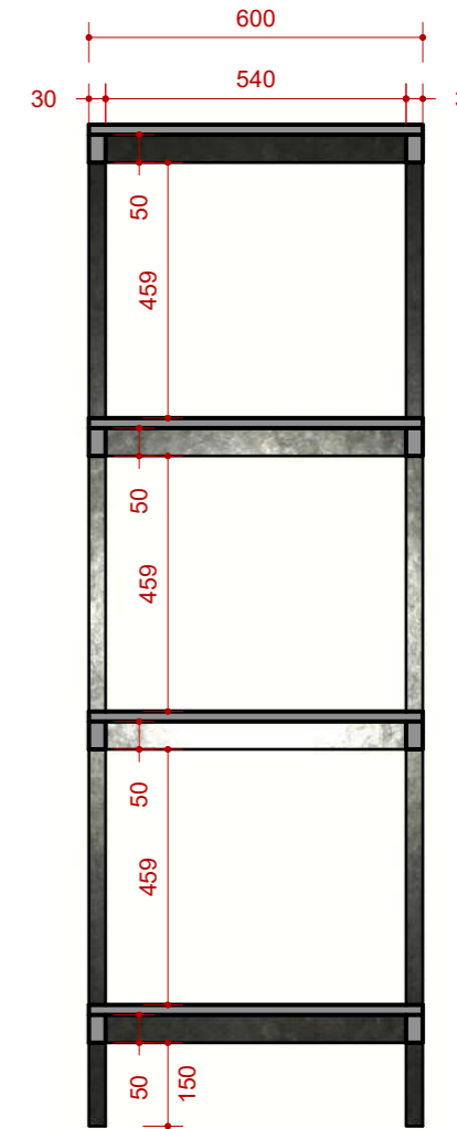
CORTE A ESCALA 1:20
